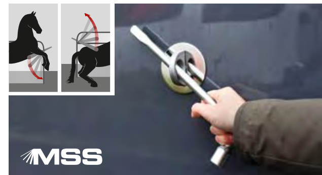
Déblocage rapide en cas d'urgence grâce au système anti-panique éprouvé à barres de sécurité Multi Safe (MSS) Peut être débloqué à l'avant et à l'arrière. La clé de roue fait partie de l'équipement de série.
